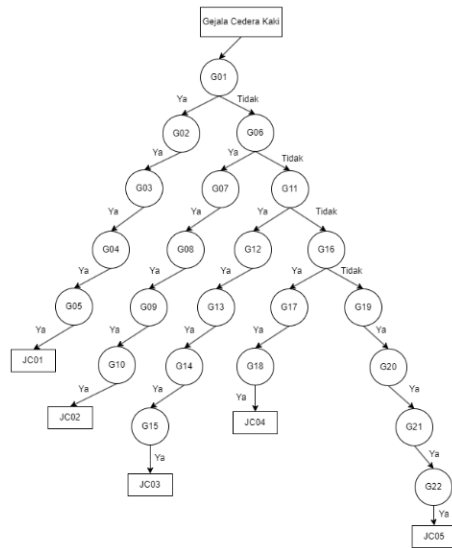
Gambar 1. Pohon Keputusan
