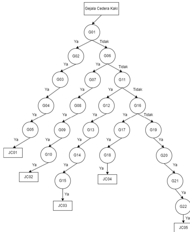
Gambar 1. Pohon Keputusan
